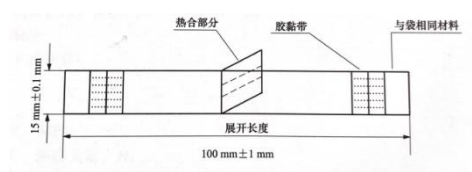
图 2 形状与尺寸
